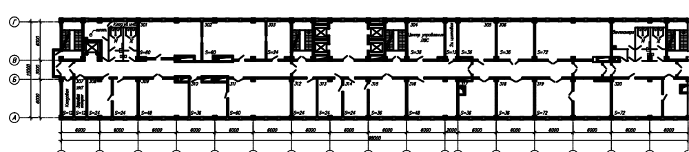
План 2 - во этажа
