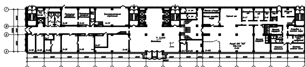
План цокольного этажа
